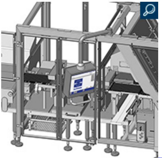
Rohschinken-Schneidelinie Interleaver
