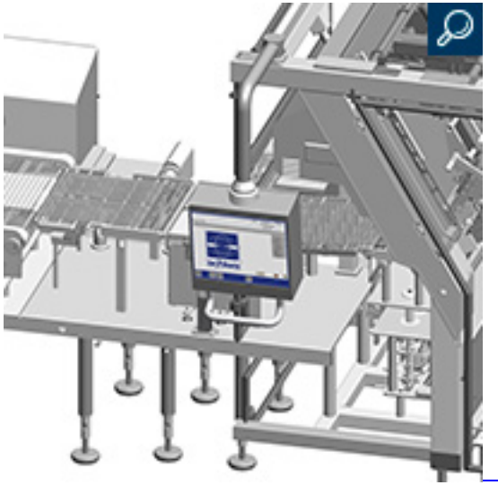
Käse-Schneidelinie
